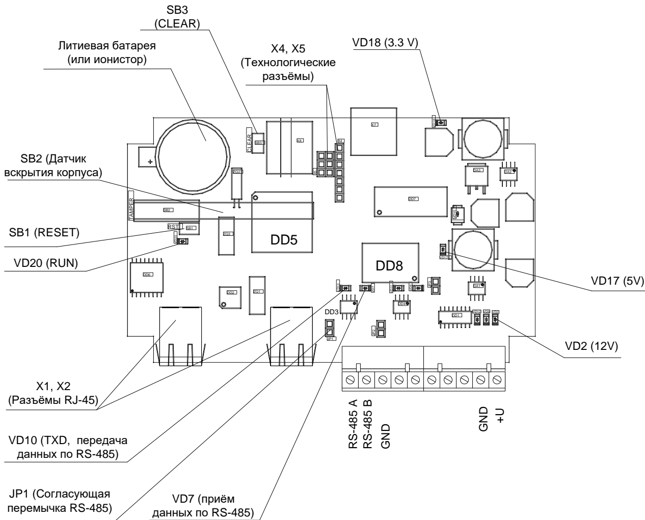
Рисунок 1. Схема расположения элементов КСК Elsys-MB-Net II
